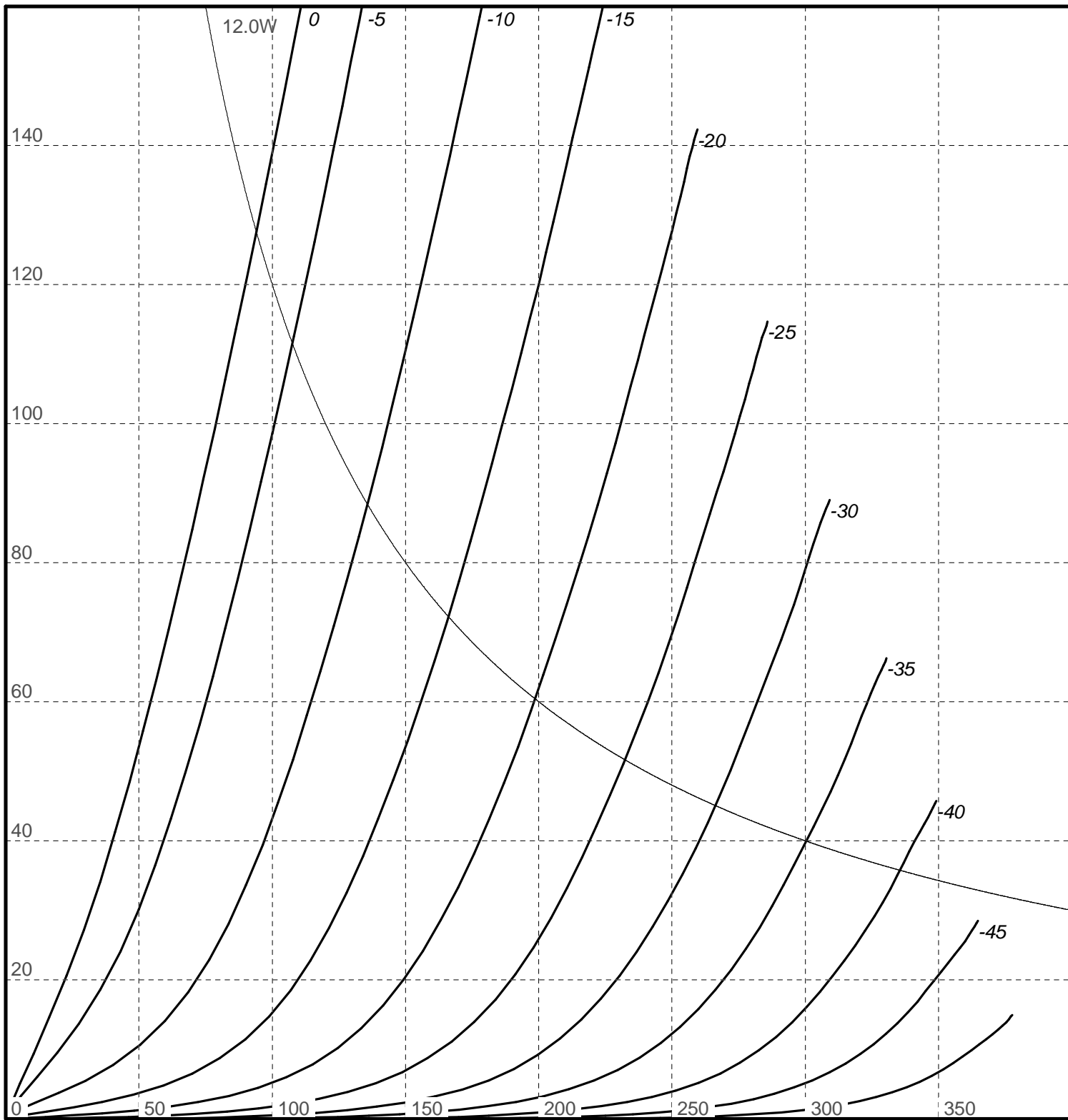
EL86 Triode. Mu=8, Rp= 1K
